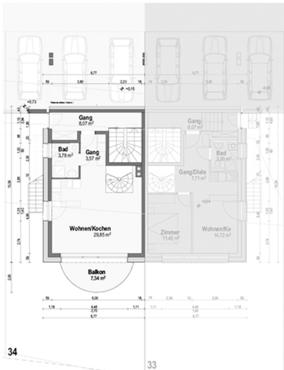
GRUNDRISS EBENE - 1
